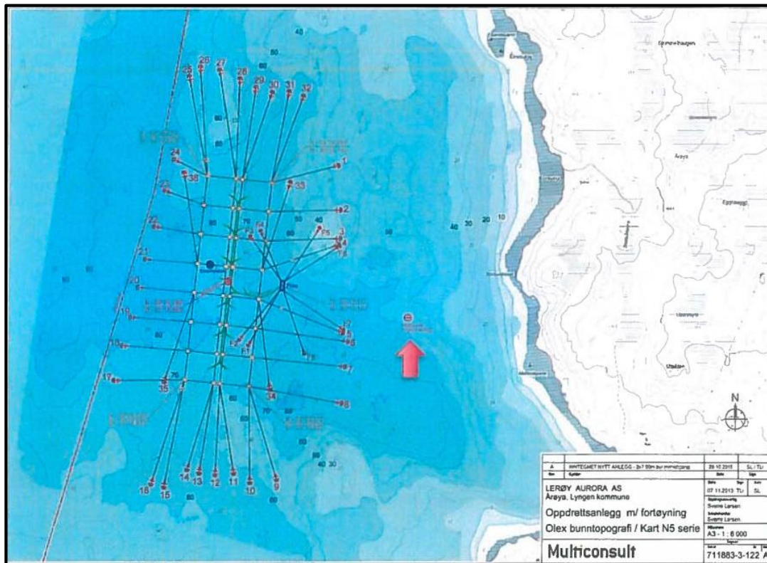
Fig. 1 – Kartutsnitt som viser ønsket plassering med fortøyninger. Senterposisjon for eksisterende anlegg er merket med rød pil.
